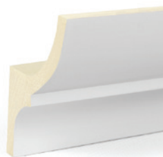
KF 701 | 70x40mm
