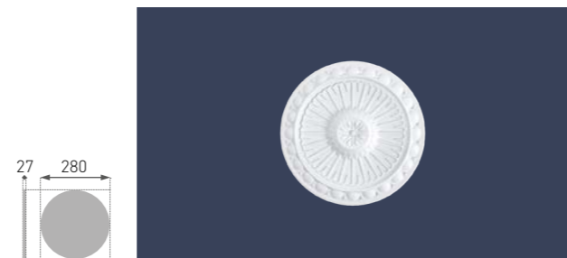
R-16 | Ø 280 mm | 5 szt.
