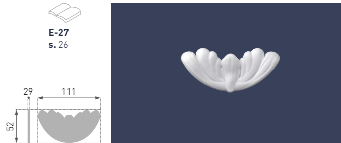
LE-27-01 | 111x52 mm | 4 szt. | 64 szt.
